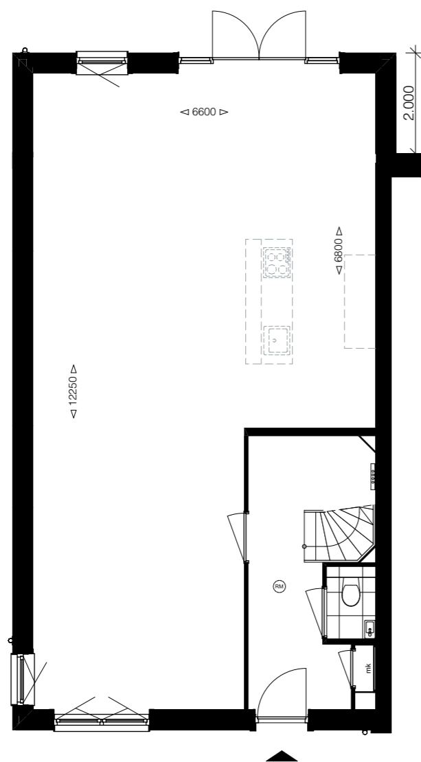
Woningtype 15b
