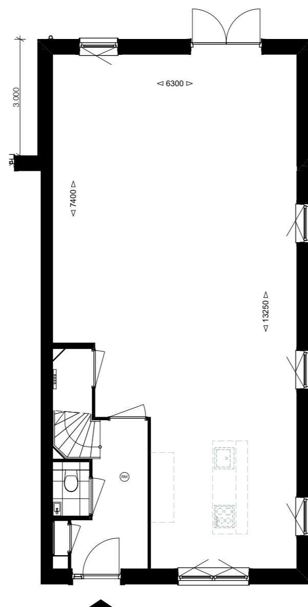
Woningtype 9b
