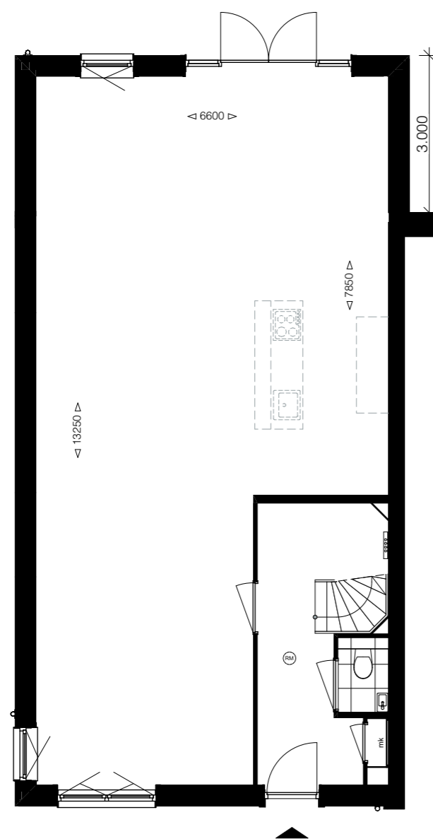
Woningtype 15b
