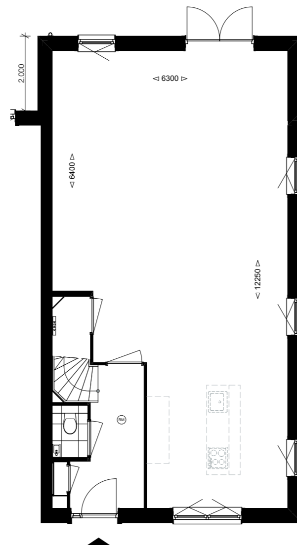
Woningtype 9b
