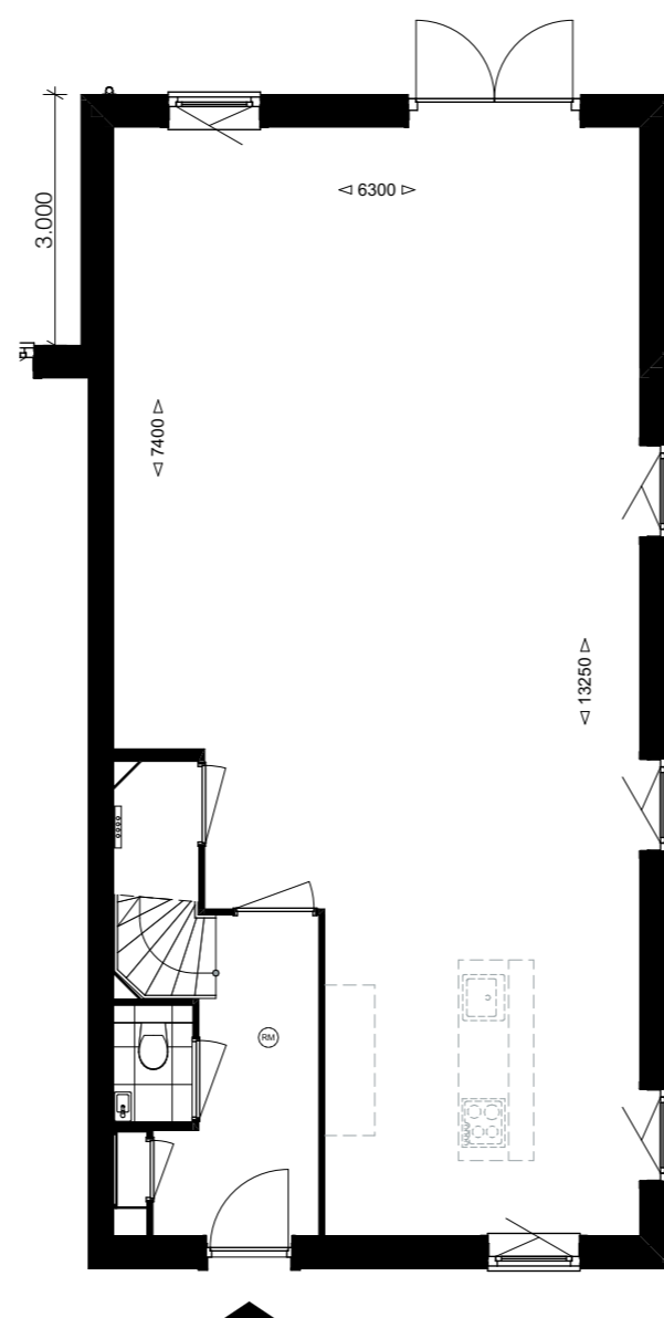
Woningtype 12b
